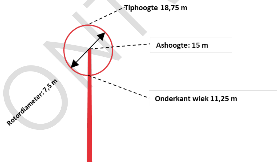
Figuur 3: Schematische weergave kleine windmolen
