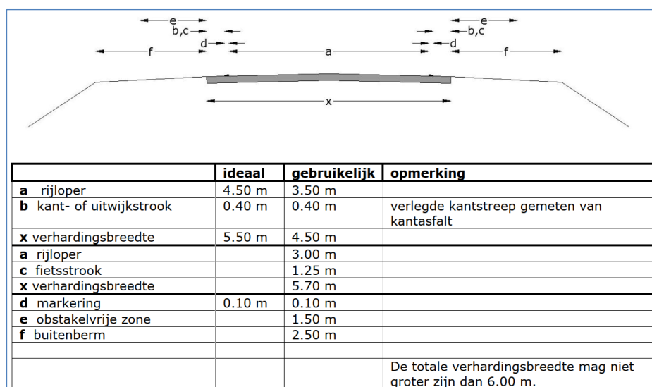
Figuur 3 – Dwarsprofiel ETW 1 [bron: Algemeen Programma van Eisen Inrichting Wegen , § 3.1.1.3]
